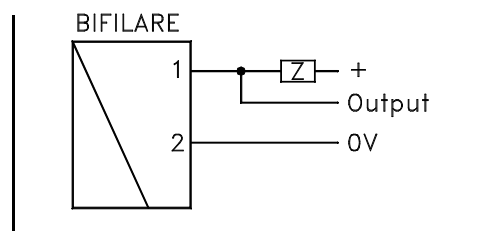
BIFILARE = Z
